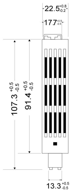
俯视图
